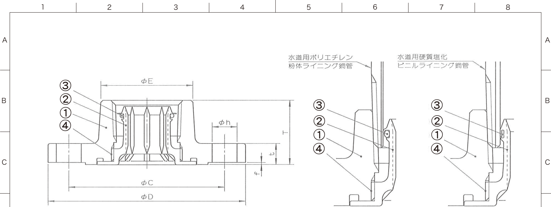
水道用ライニング鋼管接続図
